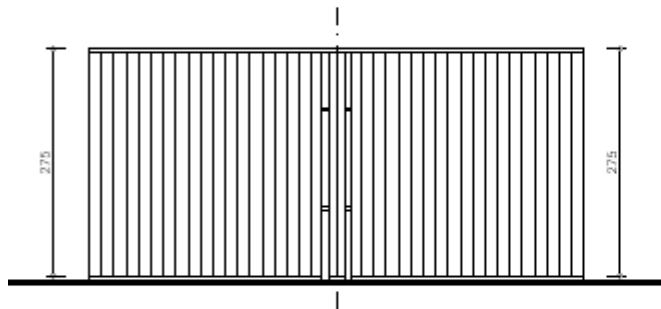
VOORGEVEL tuinberging type 1
