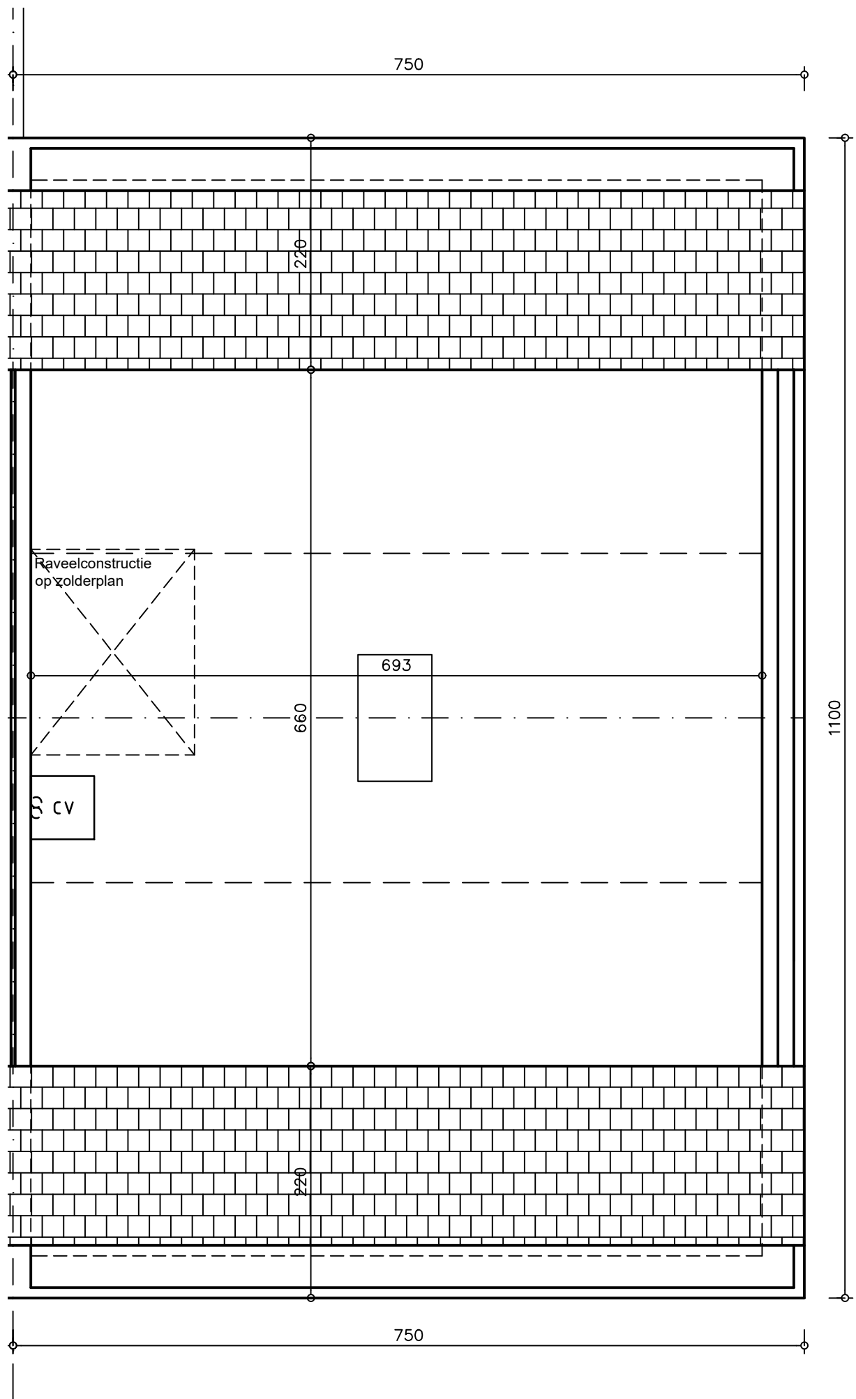
WONING 05 ZOLDER
