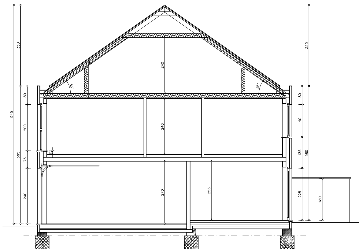
DOORSNEDE
