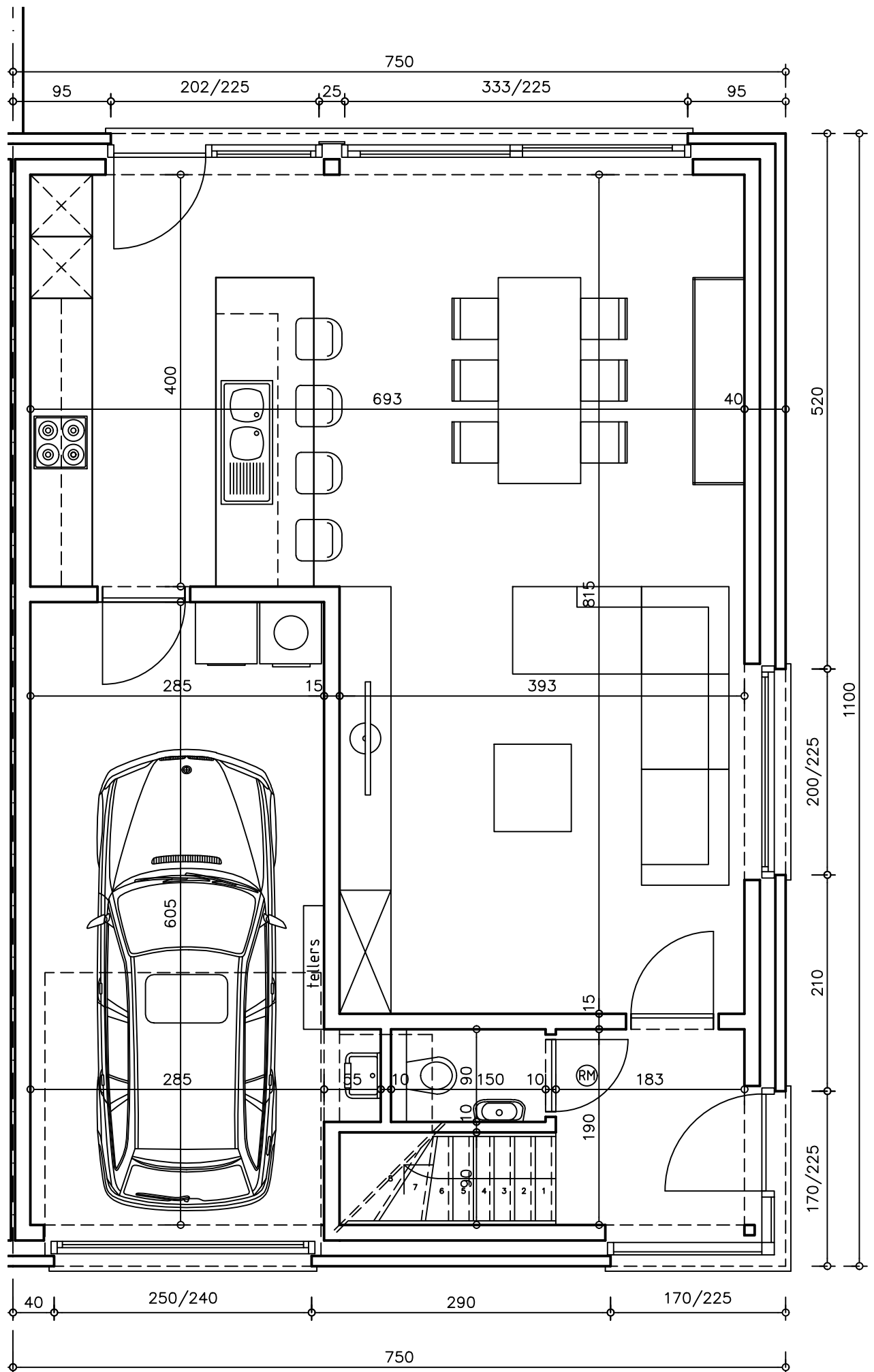
WONING 05 GELIJKVLOERS
