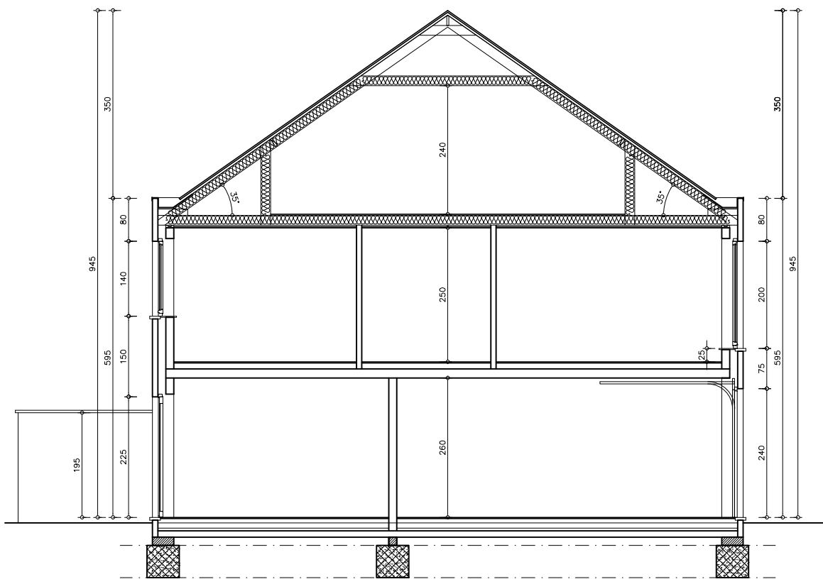
DOORSNEDE
