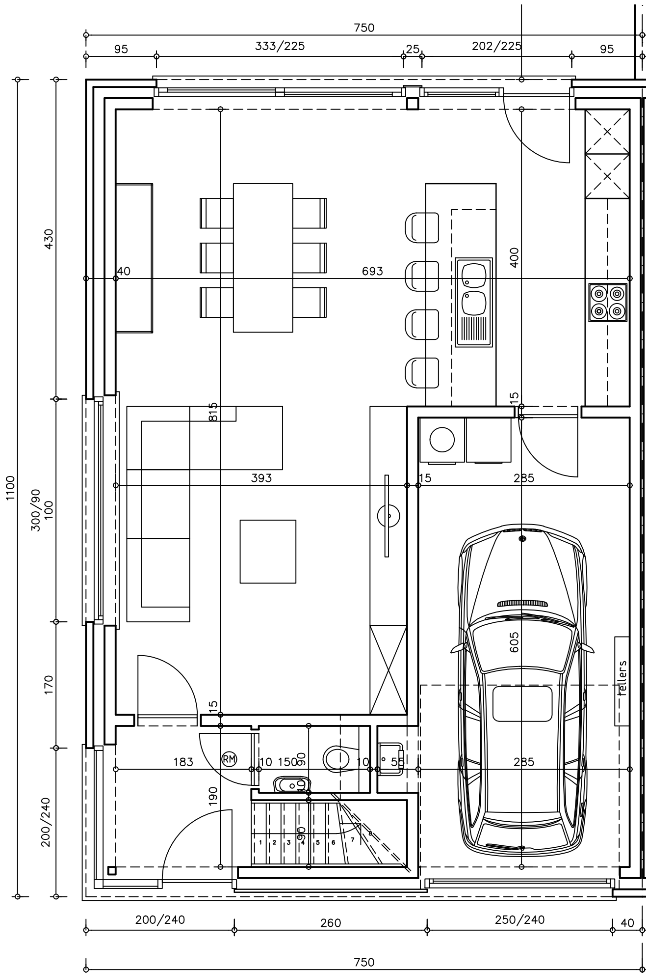
WONING 04 GELIJKVLOERS
