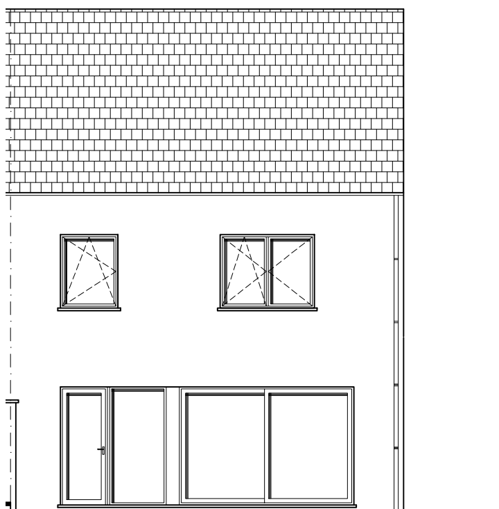
WONING 04 ACHTERGEVEL
