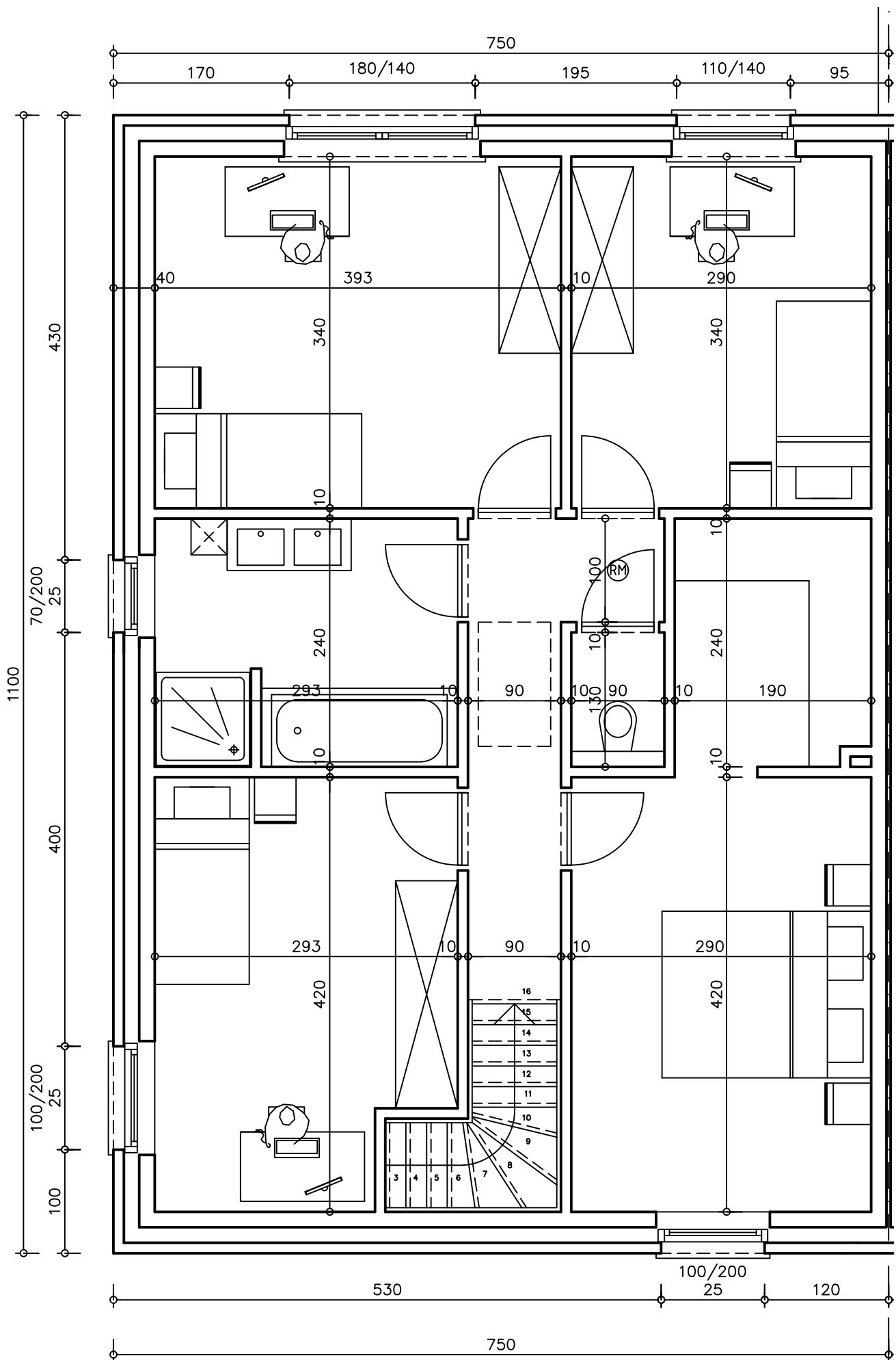
WONING 04 VERDIEPING
