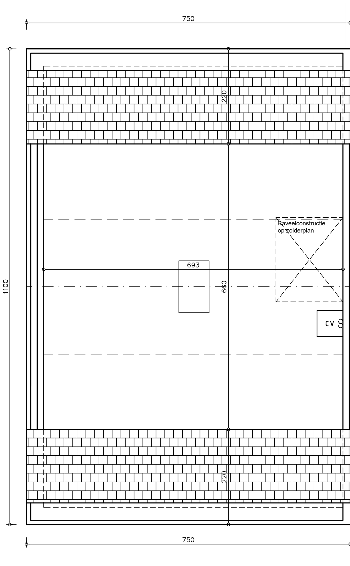
WONING 04 ZOLDER
