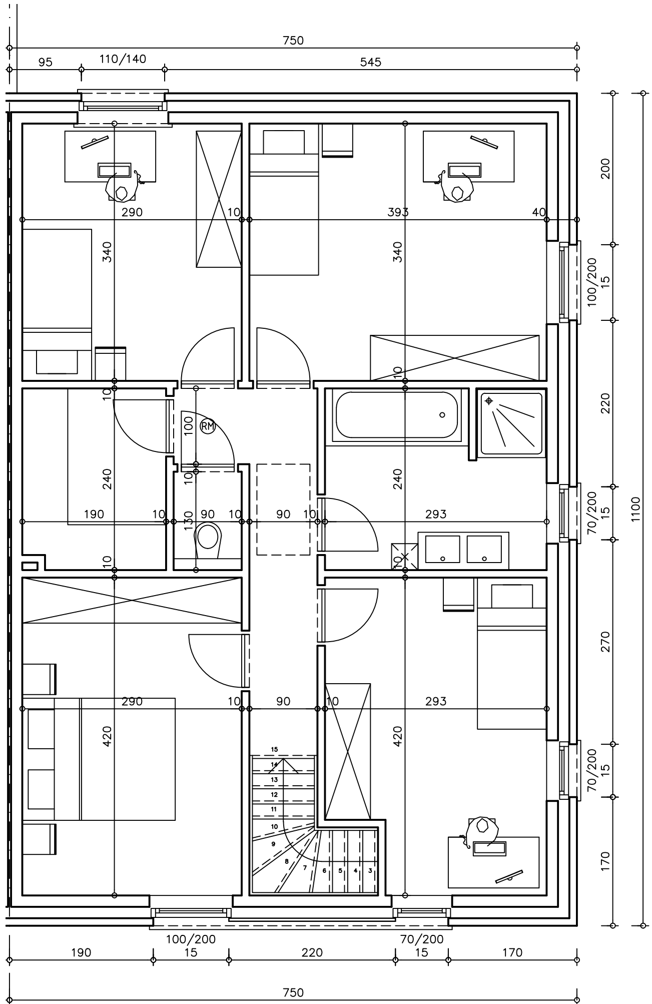
WONING 05 VERDIEPING
