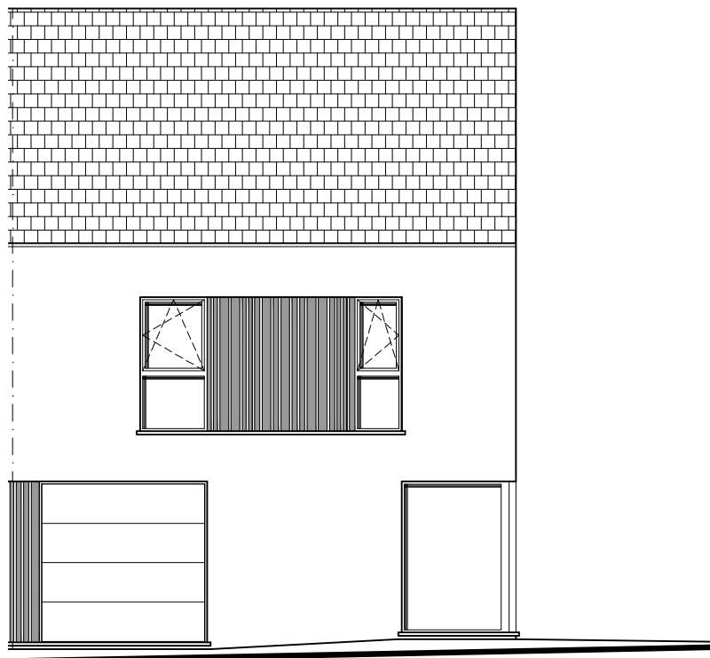
WONING 05 VOORGEVEL
