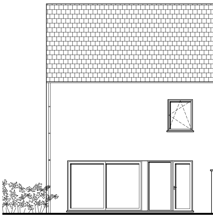
WONING 05 ACHTERGEVEL
